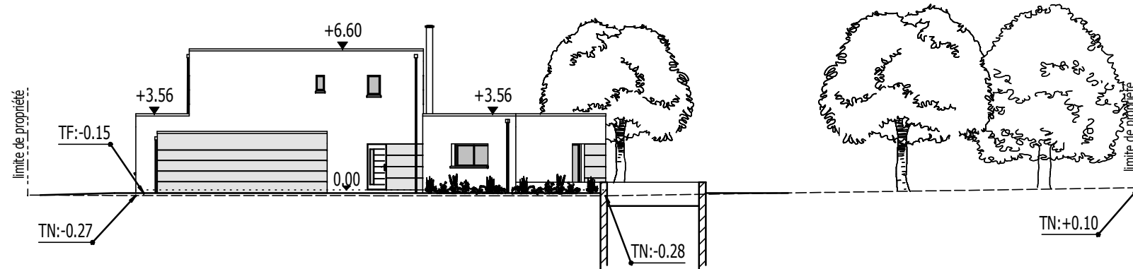
COUPE A SUR TERRAIN
