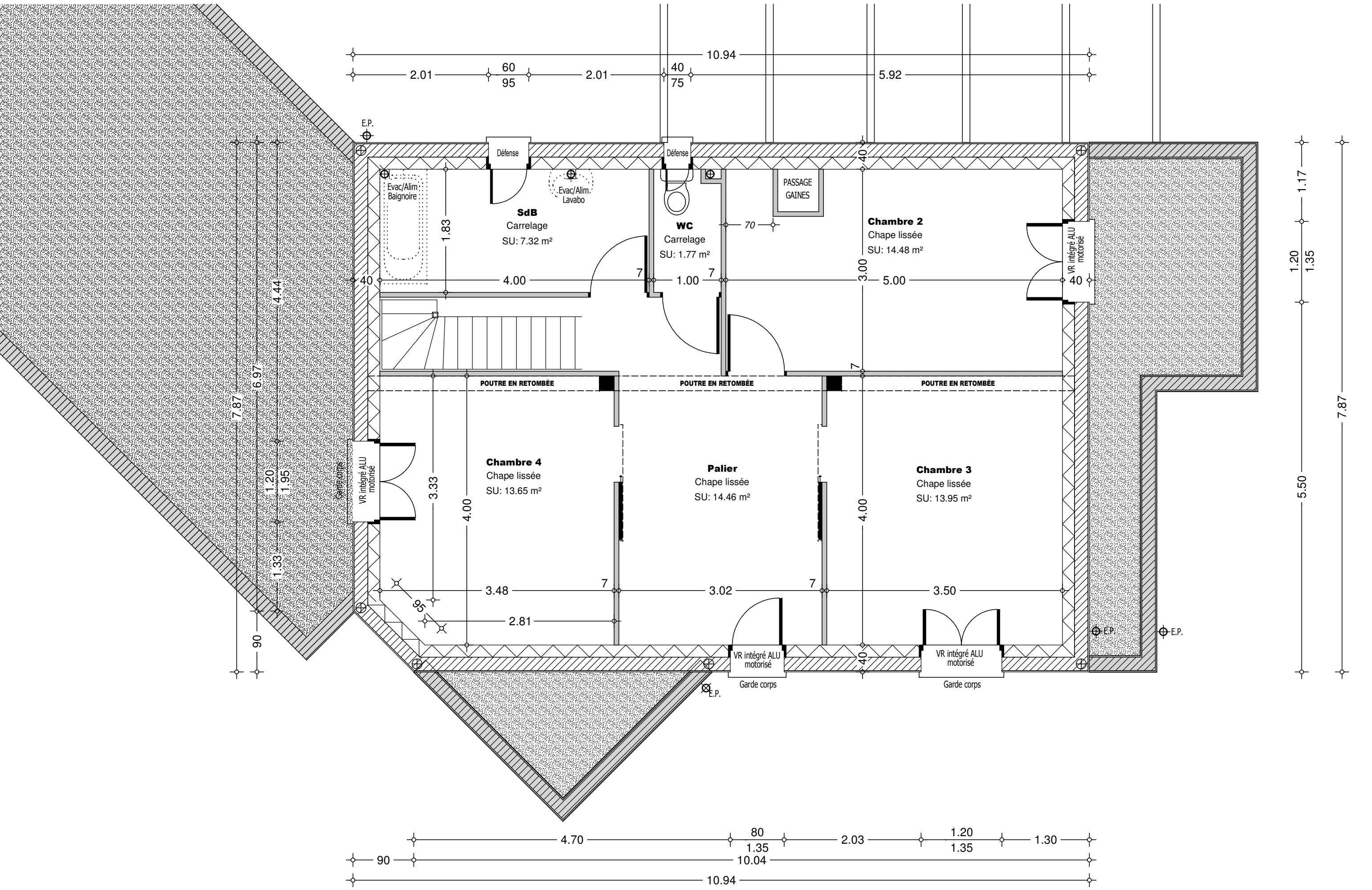
ETAGE 1/50
